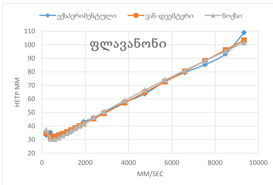
ნახ. 44: ექსპერიმენტული, ვან-დეემტერისა და ნოქსის მრუდები მოძრავი ფაზის სიჩქარის თეორიული თეფშების სიმაღლეზე დამოკიდებულების შესახებ ფლავანონისთვის.
