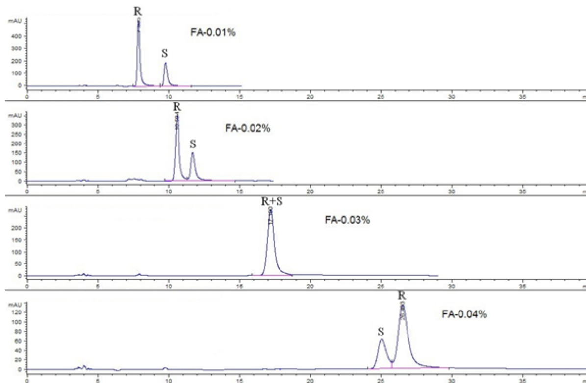
ნახ. 12: ამლოდიპინის ენანტიომერების ელუირების თანმიმდევრობას ცვლილება ცელულოზა ტრის(4-ქლორ-3-მეთილფენილკარბამატის) შემცველ სვეტზე ჭიანჭველამჟავის კონცენტრაციის გაზღვრით აცეტონიტრილში [147-148]
