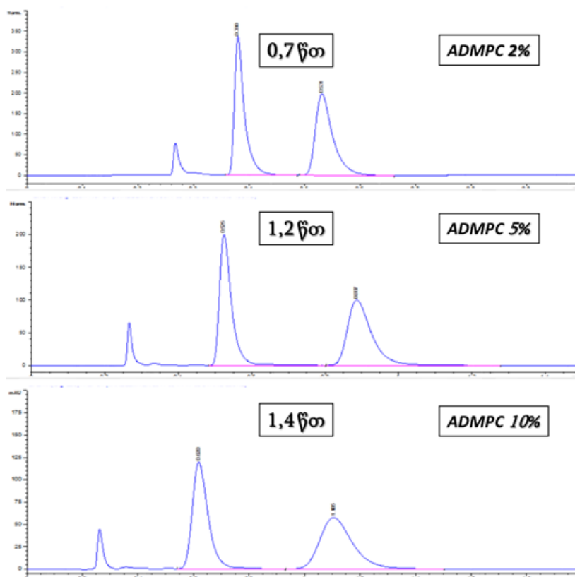
ნახ. 40: ფლაგანონის ენანტიომერების ანალიზი 5,0 მლ/წთ სიჩქარეზე.
