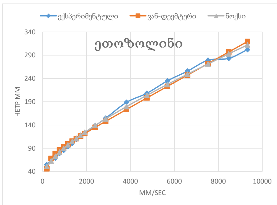
ნახ. 43: ექსპერიმენტული, ვან-დეემტერისა და ნოქსის მრუდები მოძრავი ფაზის სიჩქარის თეორიული თეფშების სიმაღლეზე დამოკიდებულების შესახებ ეთოზოლინისთვის.
