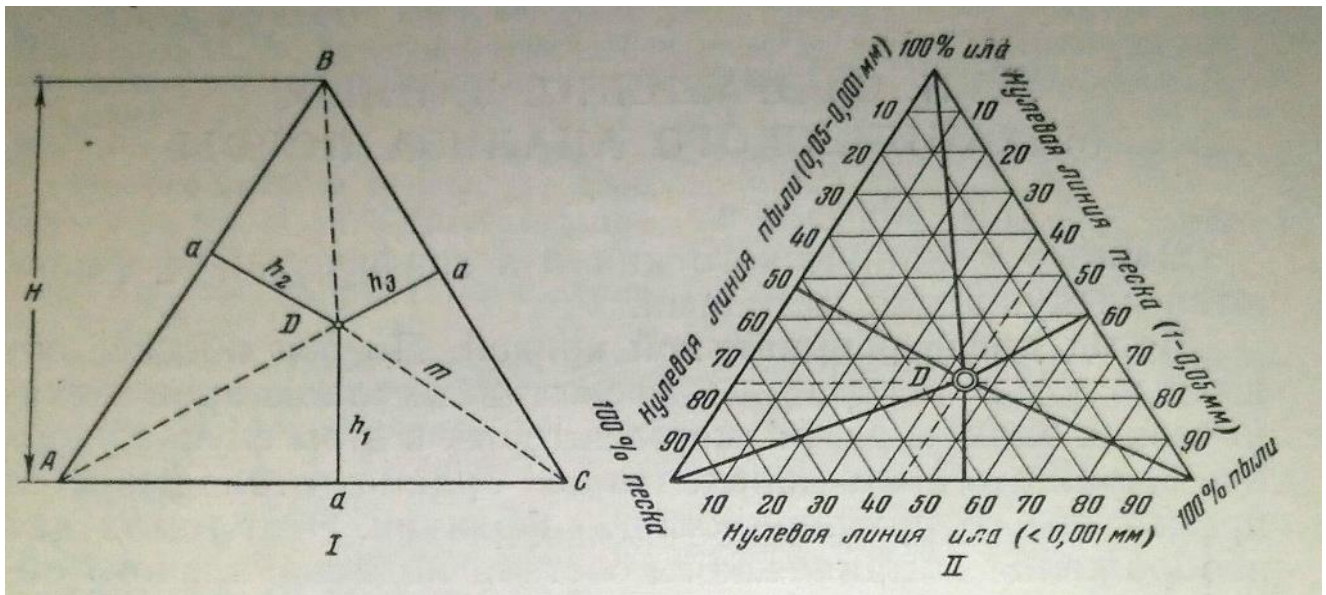
ნახ. 26. ნიადაგის გრანულომეტრიული შედგენილობის გამოსახვა გიბს-როაზომის სამკუთხედის მიხედვით
