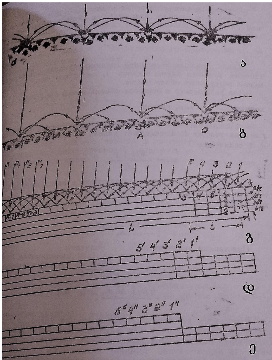
ნახ. 19. წვიმის წვეთების ნიადაგზე მოქმედების სქემები: ა-წვიმის წვეთების დაცემის და ნიადაგის ჰორიზონტალურ ზედაპირზე ნიადაგის ნაწილაკების გაშეფების სქემა; ბ-წვიმის წვეთების დაცემის და ნიადაგის დახრილ ზედაპირზე ნიადაგის ნაწილაკების გაშეფების სქემა; გ-წვიმის წვეთების დაცემის და ნიადაგის ნაწილაკების ფერდობის დახრილობის მიმართულებით მოძრაობის სქემა; დ, ე-წვიმის წვეთების დარტყმით ნიადაგის ფენის თანდათანობით მოხსნა; 1, 2, 3, 4, 5-წვეთების ნომრები
