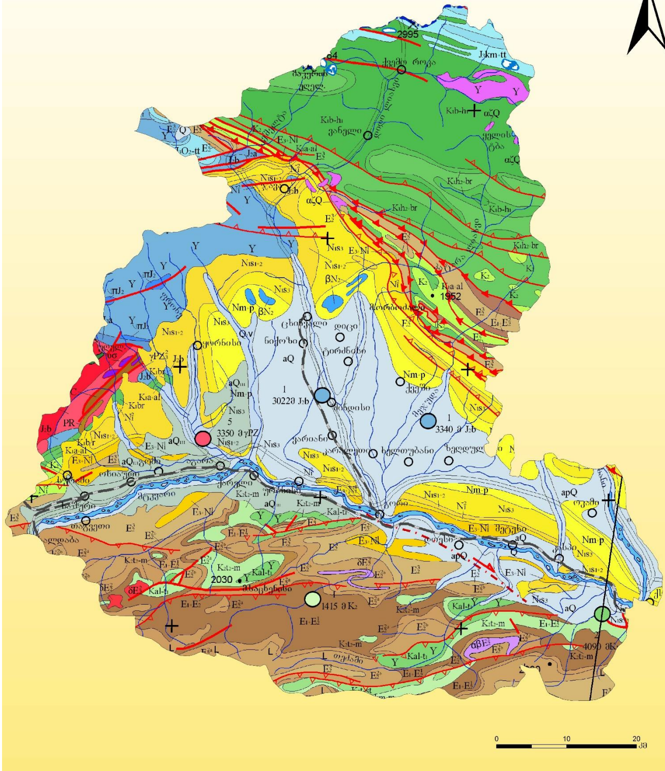
ნახ. 3. შიდა ქართლის გეოლოგიური აგებულება (გუჯაბიძე)
