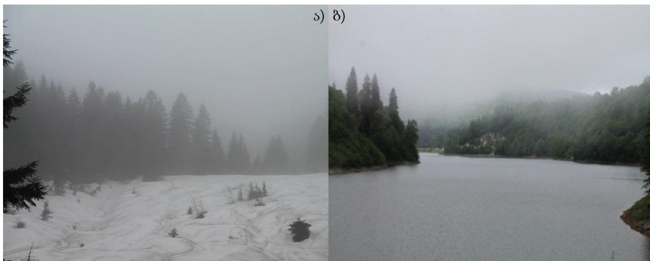
ნახ. 6. ა). ნისლის შემოსვლა ნაქერალას ტერიტორიაზე ბ). ნისლის შემოსვლა შაორის ქვაბულში
