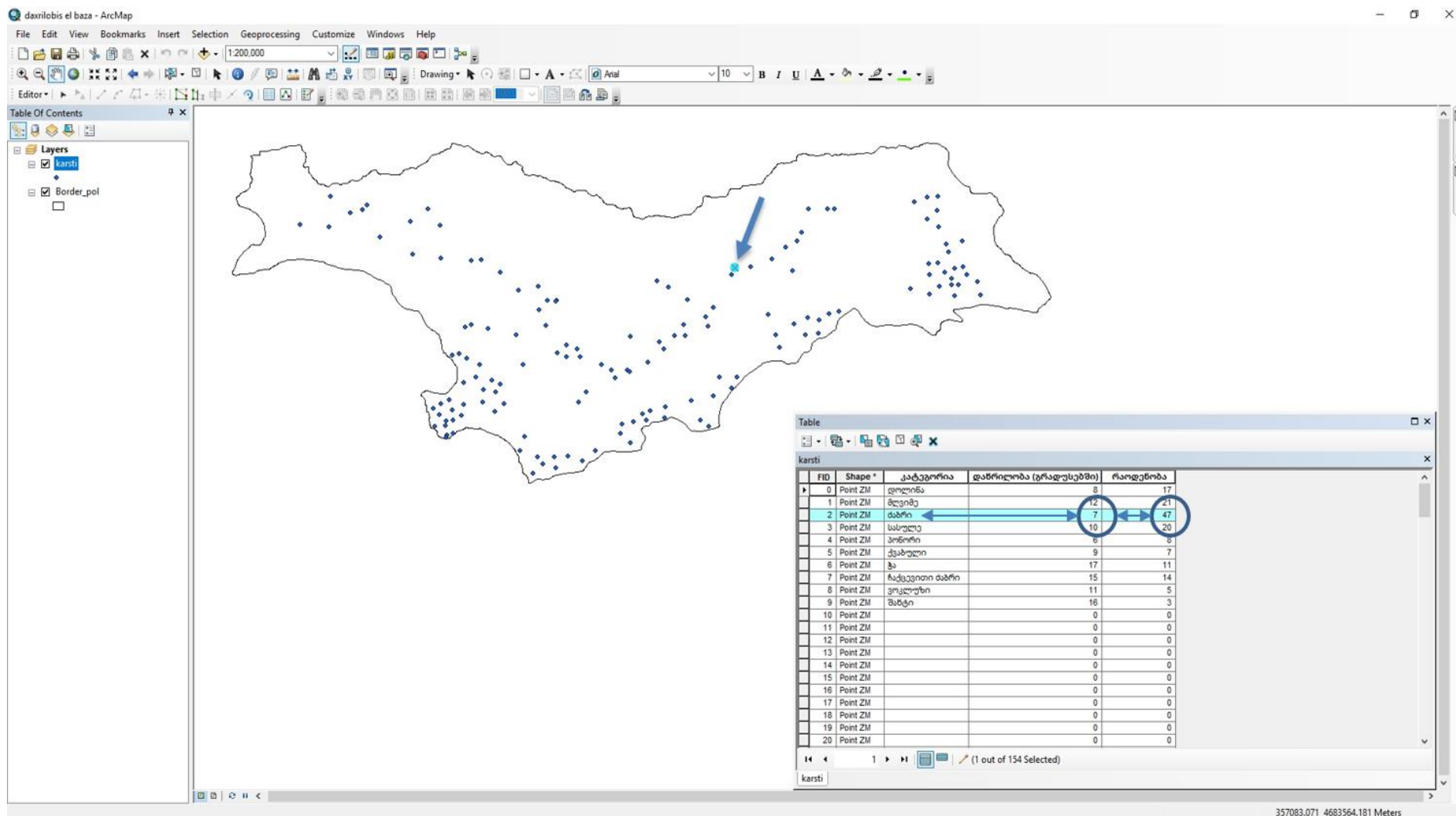
ნახ. 43. საკვლევი ტერიტორიის ფარგლებში, მოცემულ ელ. ბაზაში ასახულია სპელეო-ობიექტების (მღვიმე, დაბრი, დოლინა და სხვა) განვითარება ფერდობების დახრილობის მიხედვით (°)
