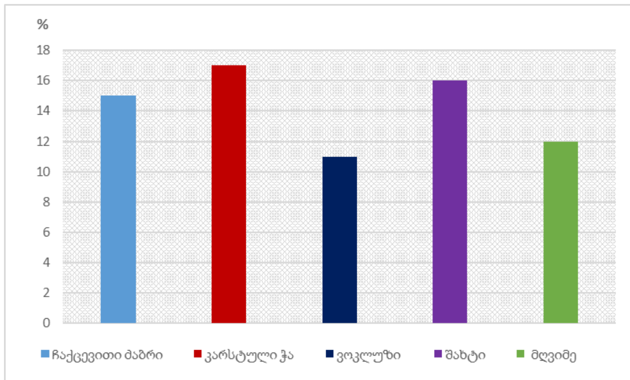
ნახ. 39. კარსტული ობიექტების გავრცელება რელიეფის დახრილობის მიხედვით ( >10^{\circ} )
