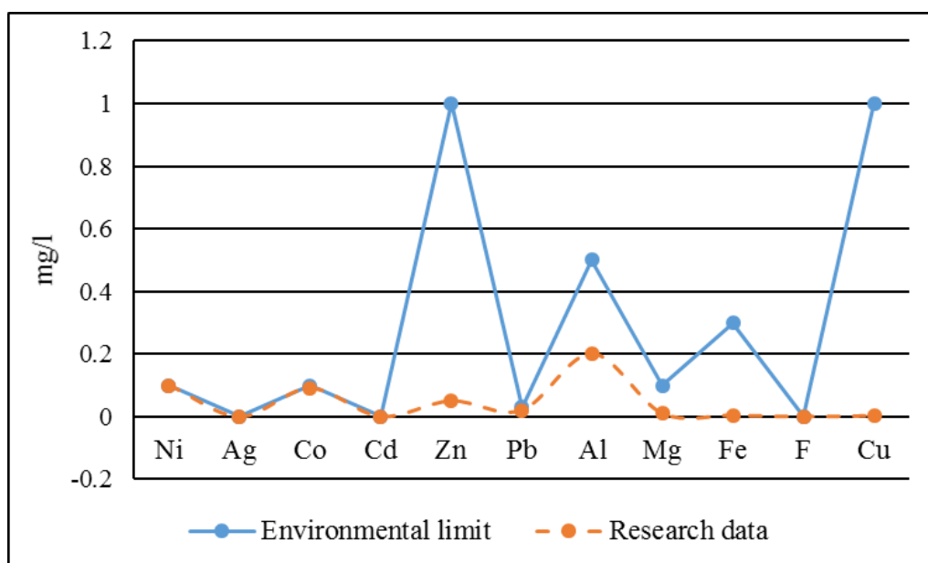
ნახ. 49. კიდობანას კარსტულ წყალში მძიმე ლითონთა კონცენტრაცია
