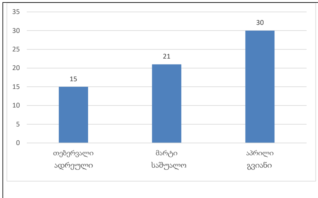
ნახ. 8. თოვლის საფარის ალების საშუალო პერიოდები თვეების მიხედვით
