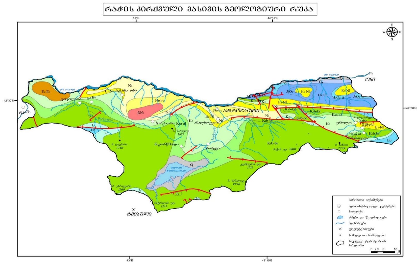
ნახ. 2. საკვლევი ტერიტორიის გეოლოგიური რუკა (ავტორი: გ. გუჯაბიძე. რედაქტორი: ე. გამყრელიძე, 2003. მასშტაბი 1:500 000)
