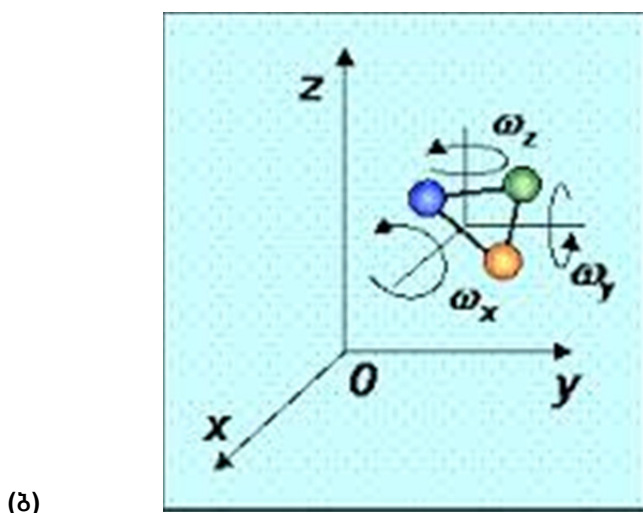
ნახ. 13. წრფივი (ა) და არაწრფივი (ბ) მოლეკულების ბრუნვითი მოძრაობები
